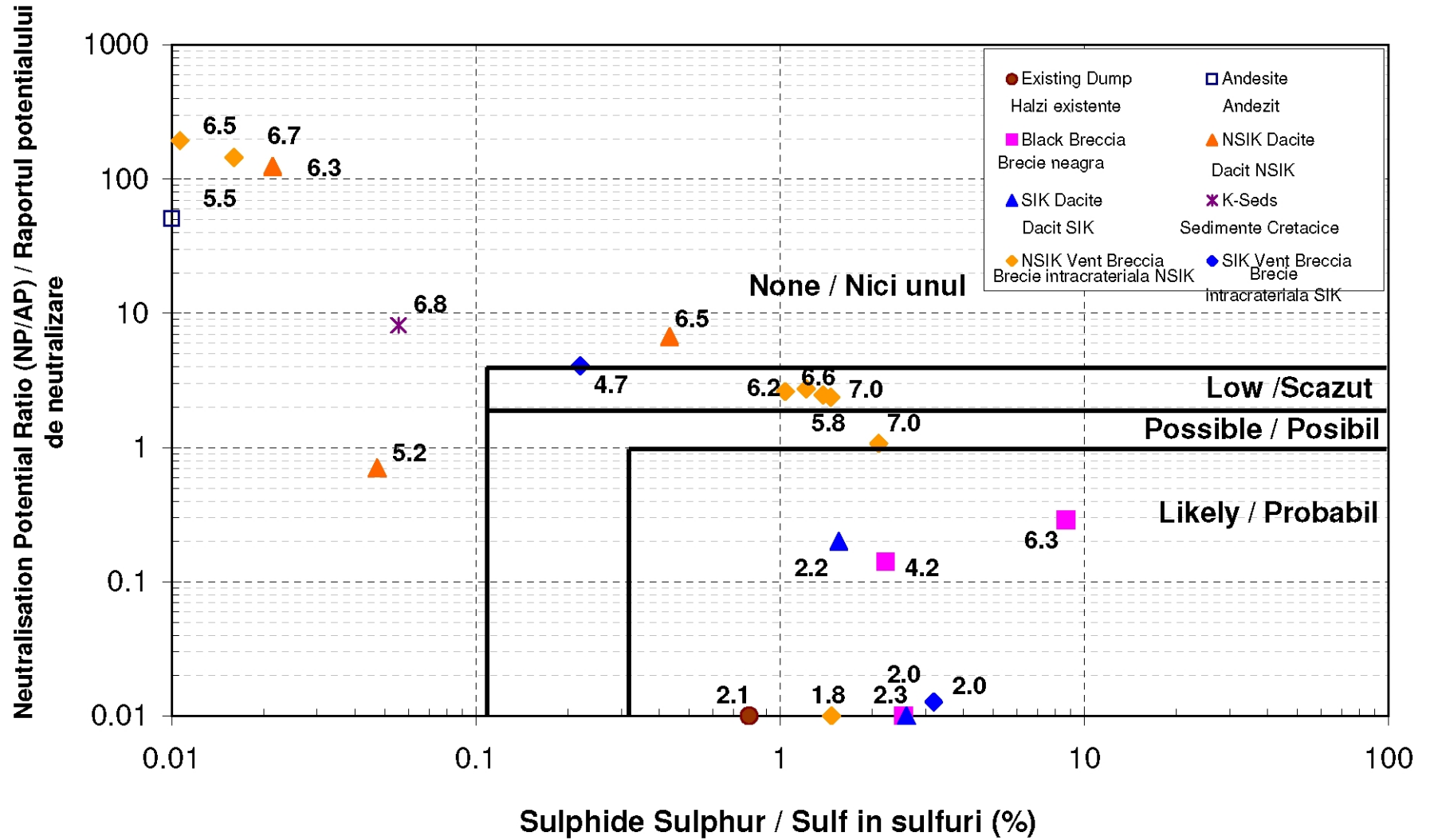
EXHIBIT / PLANSĂ 4.5.6 PLOT OF ABA DATA FOR FIELD COLUMN SAMPLES WITH LEACHATE PH ILLUSTRATED / DIAGRAMA VALORILOR DE BILANT ACID - BAZA PENTRU TESTELE DE LESIERE ÎN COLOANA EFECTUATE ÎN CONDITII DE TEREN, CU MENTIONAREA VALORILOR DE PH ALE LESIATULUI
